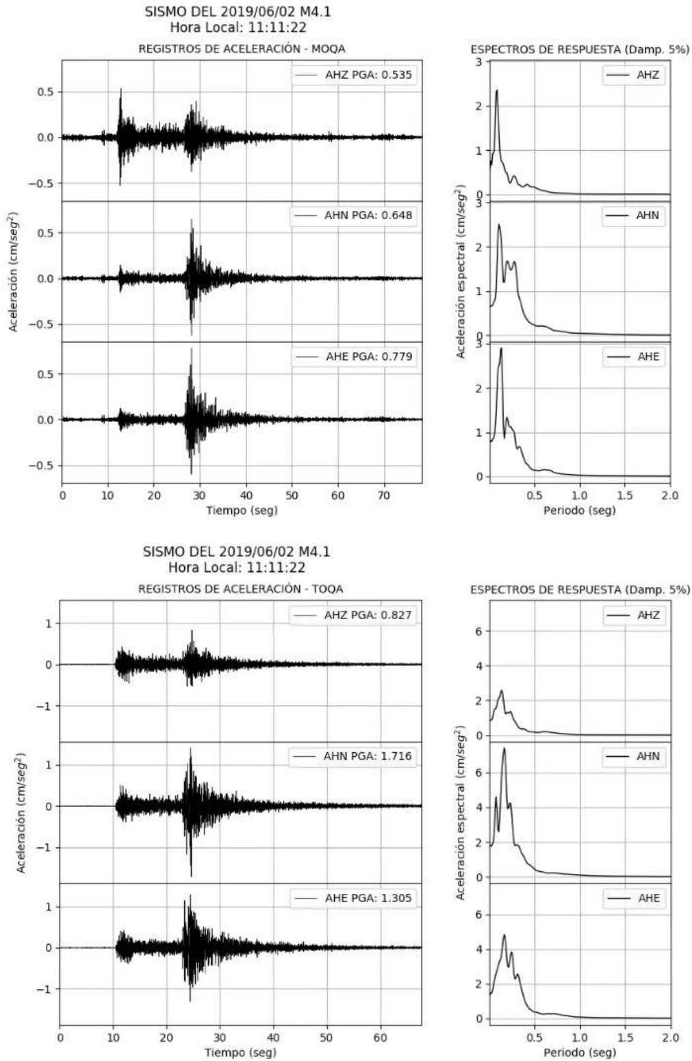
Figura 2. Registros de aceleración para el sismo del 02/06/2019. Estaciones: MOQA y TOQA.
