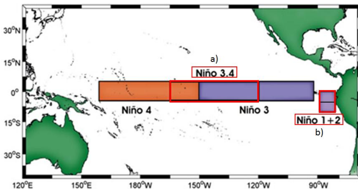
Áreas de monitoreo a) Región Niño 3.4 (5°N-5°S / 170°W-120°W) y b) Región Niño 1+2 (0°-10°S / 90°W-80°W)
